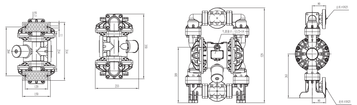
塑料/氟塑料 PP/PVDF
