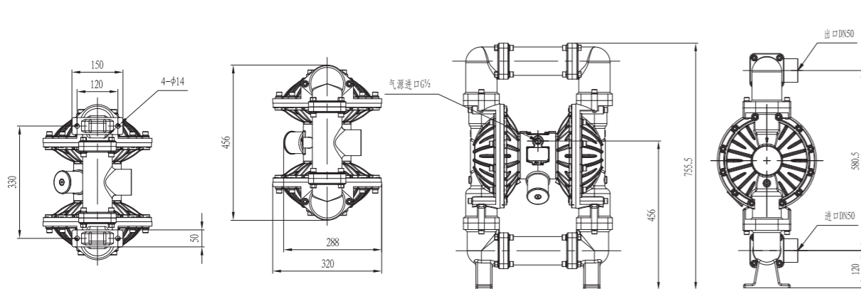
铝合金 Aluminum alloy
