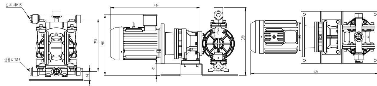
铝合金 Aluminum alloy
