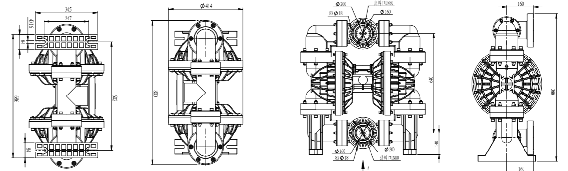
塑料/氟塑料 PP/PVDF
