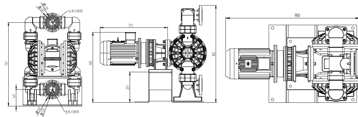
塑料/氟塑料 PP/PVDF
