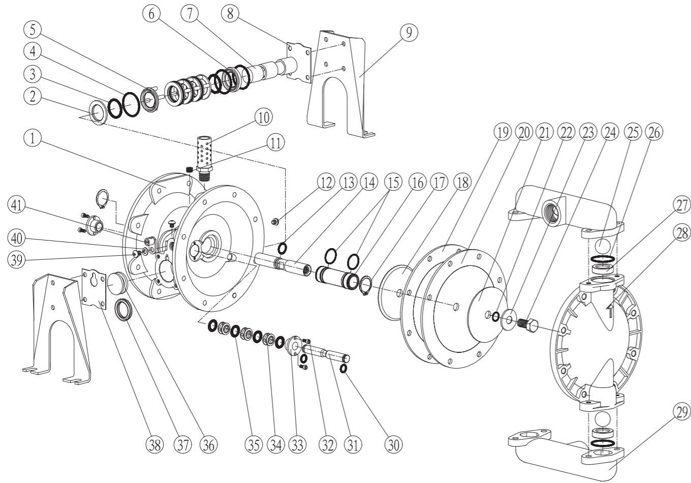
RA-25L零部件明细表
